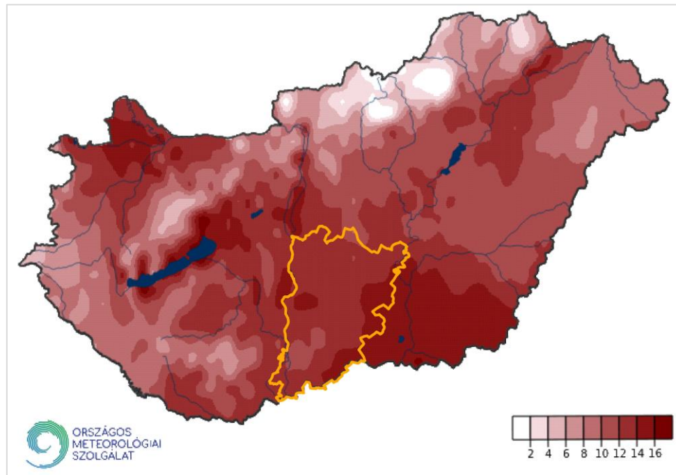
30. ábra: Hőhullámos napok (napi középhőmérséklet > 25°C) számának megfigyelt változása az 1981–2020-as időszakban
