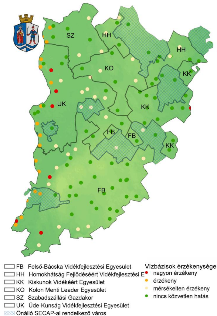
42. ábra: Ivóvízbázisok klímaérzékenysége
