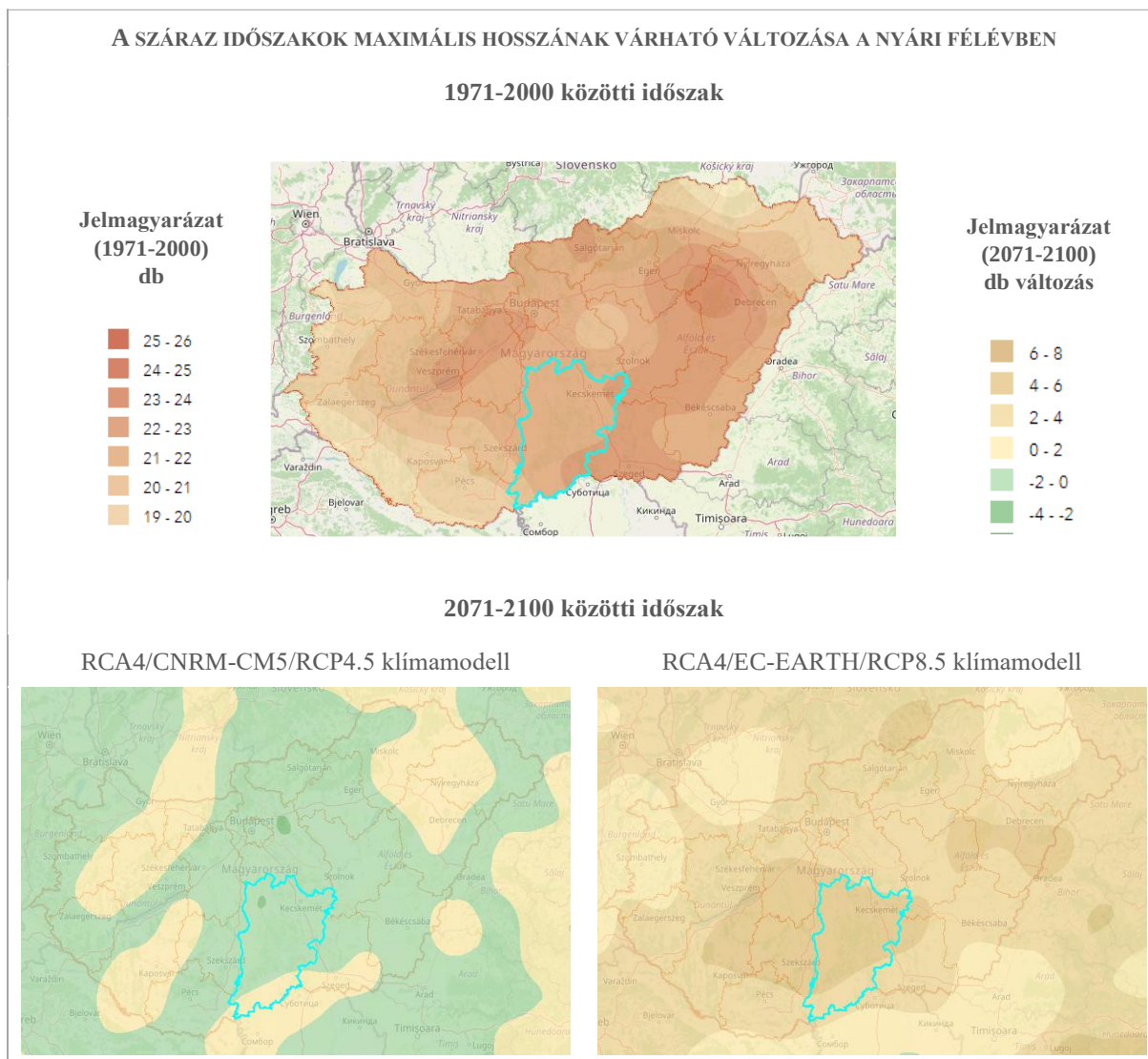
36. ábra: A száraz időszakok maximális hosszának változása a nyári félévben
