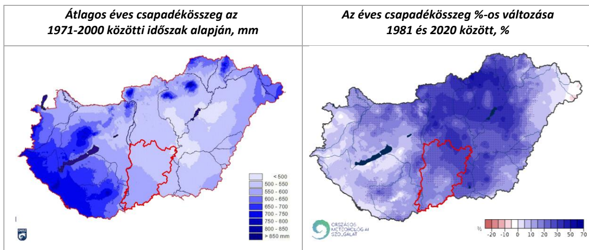
32. ábra: Éves csapadékösszeg és változásának alakulása az elmúlt 50 évben
