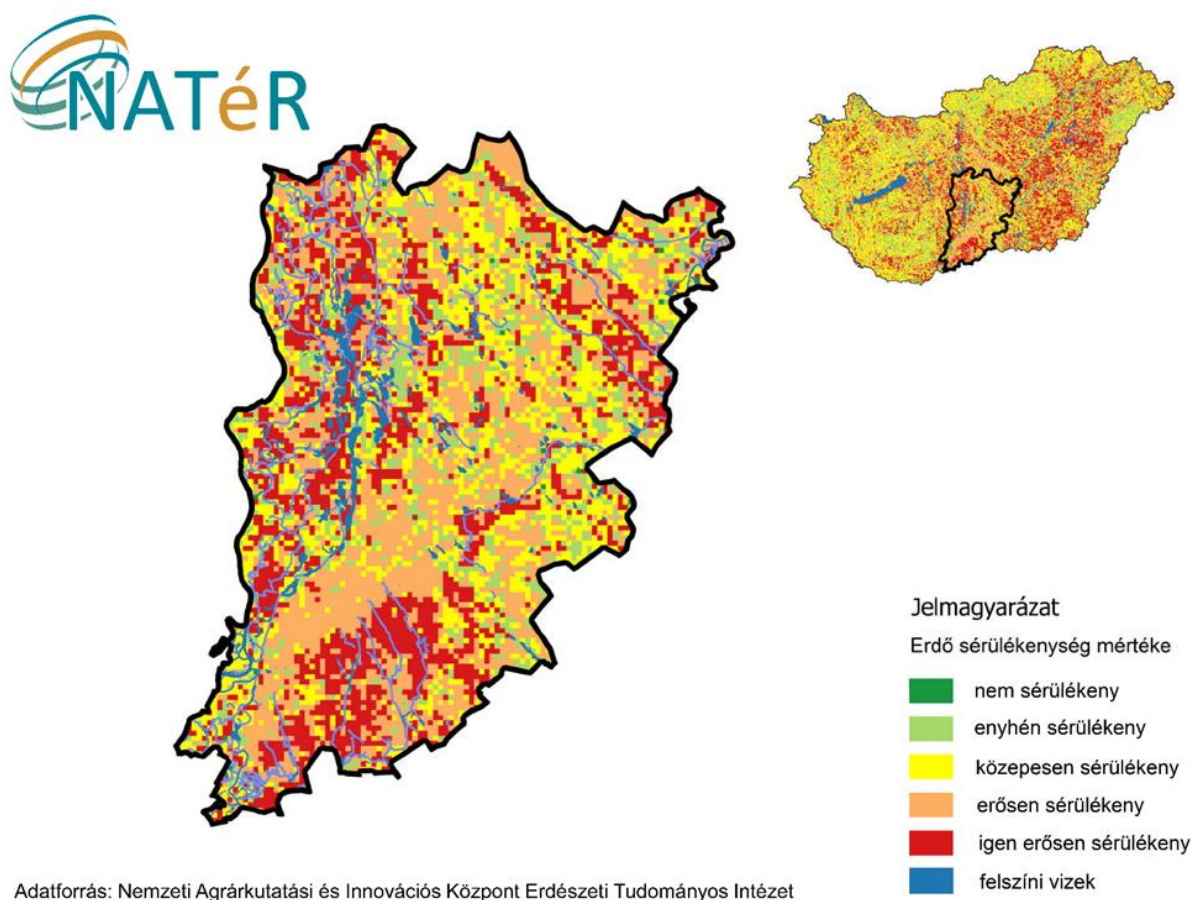
45. ábra: Erdők összesített sérülékenysége a vármegye területén
