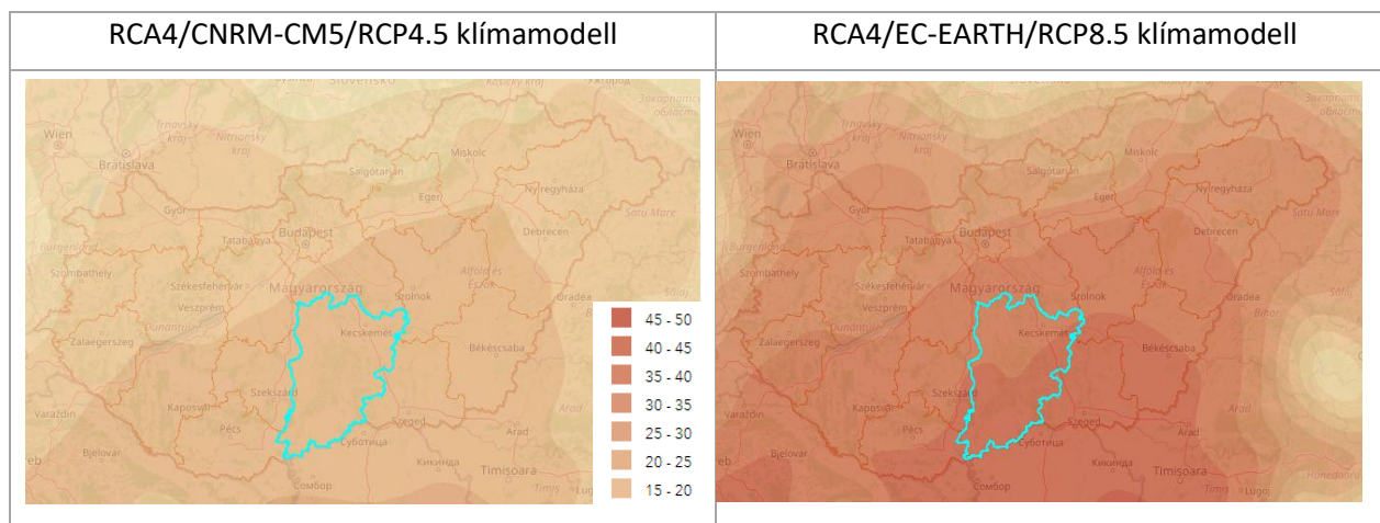
31. ábra: Hőhullámos napok (napi középhőmérséklet > 25°C) átlagos évi számának várható változása 2071-2100 közötti időszakban az 1971-2000-es időszakhoz képest (nap)
