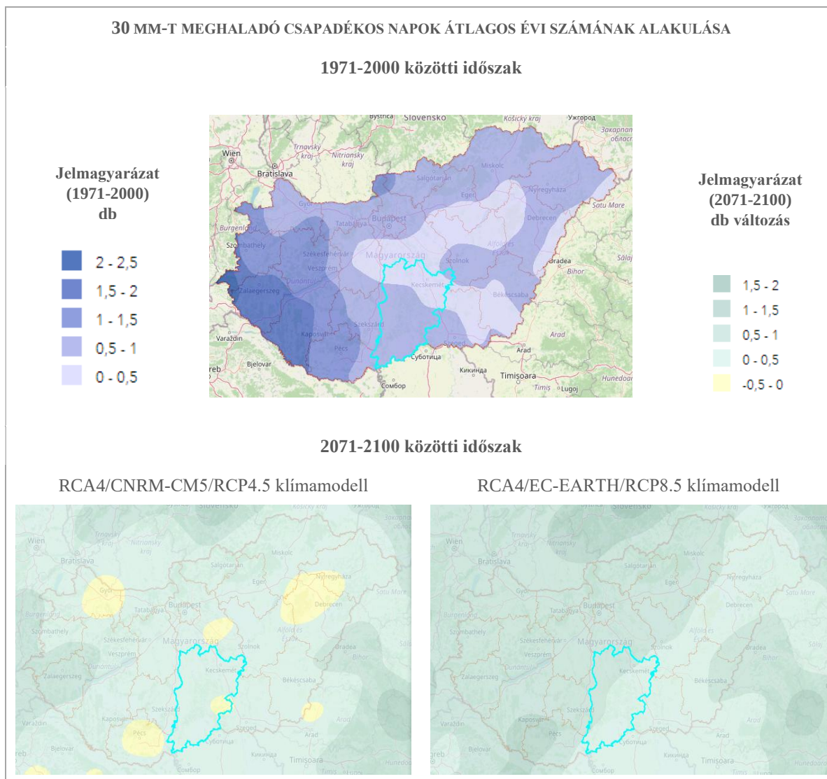
35. ábra: 30 mm-t meghaladó csapadékos napok átlagos számának várható változása, 2071-2100 (nap)
