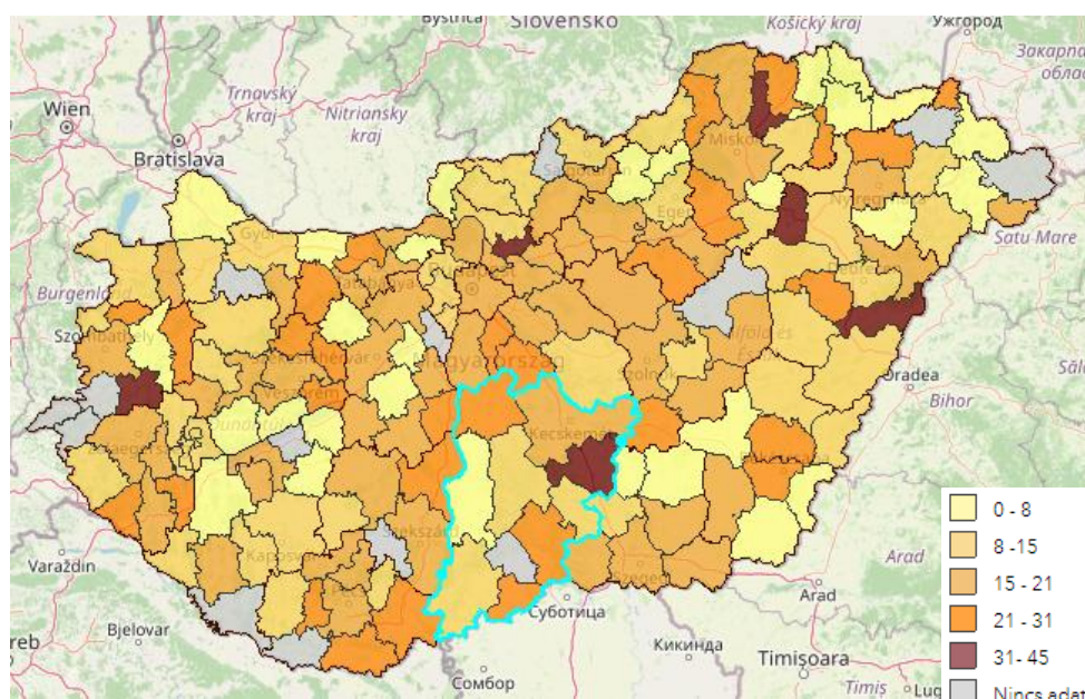
37. ábra: Hőségnapokhoz kapcsolódó többlethalálozás, 2005-2014 (%)
