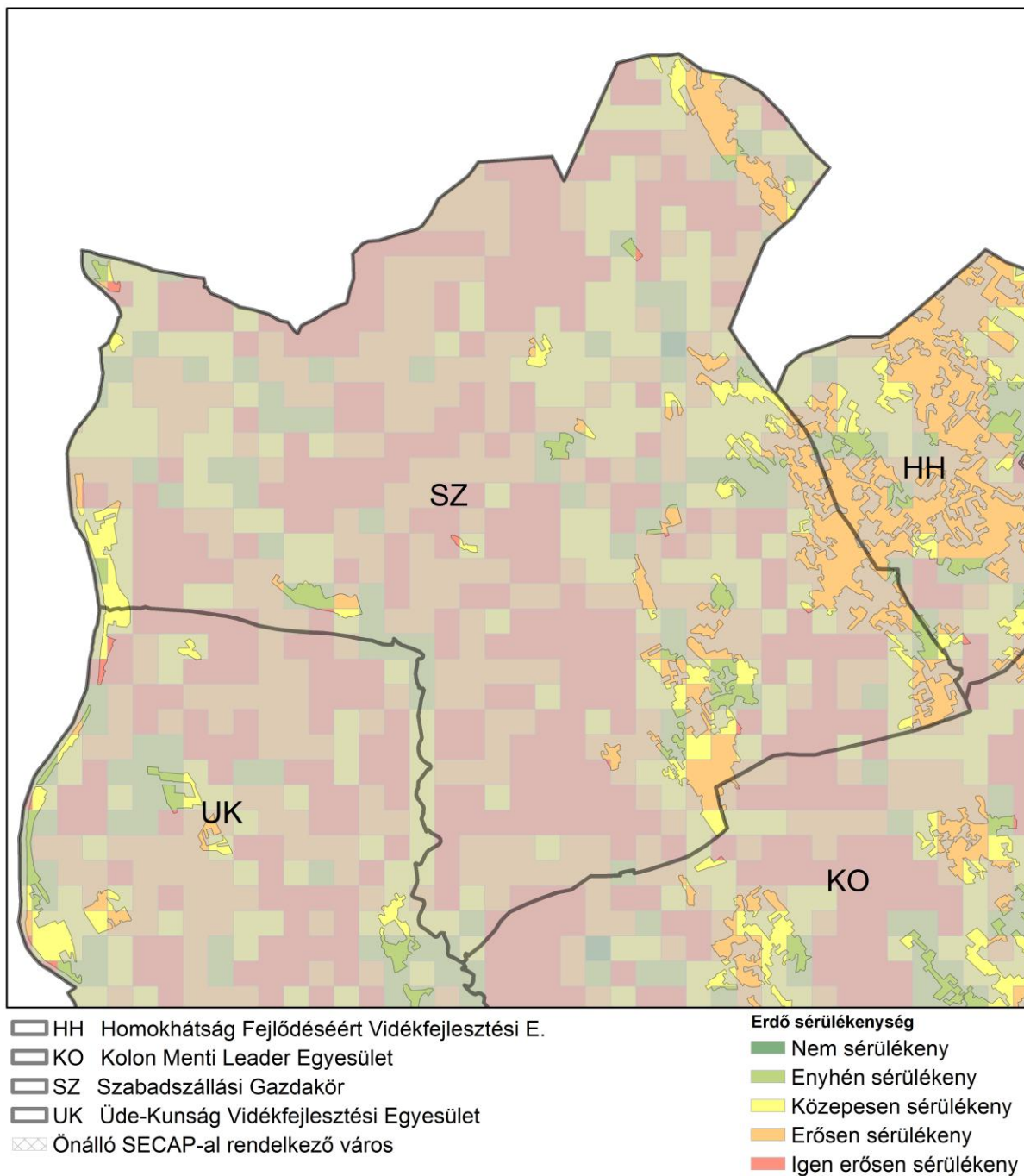
47. ábra: Erdészeti sérülékenység az egyesület területén, kiemelve az erdős, cserjés borítású területek
