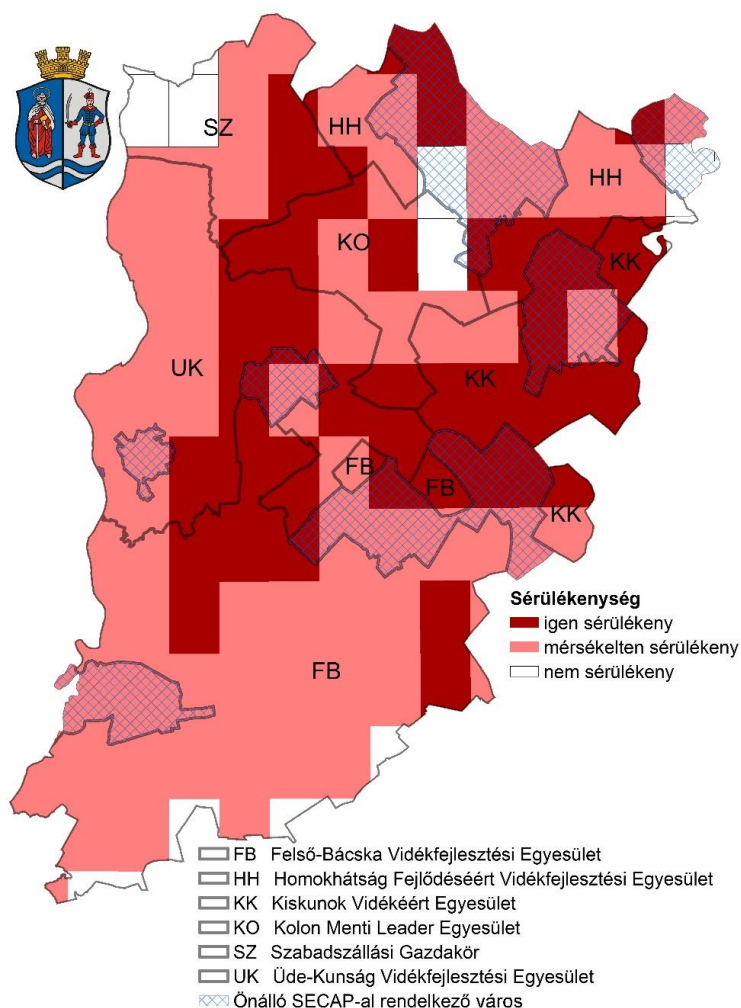
44. ábra: Tavasz vetésű növények sérülékenysége
