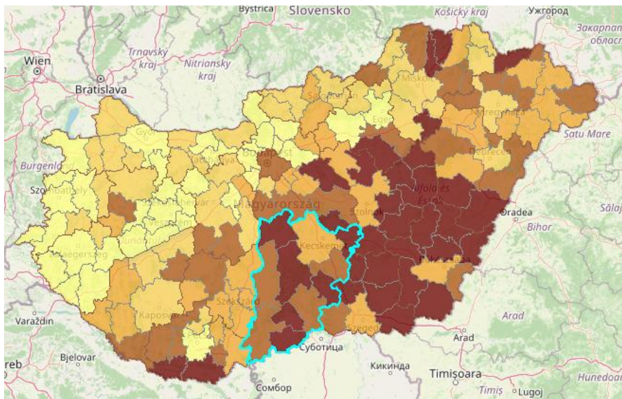
39. ábra: Hőhullámok hatásaival szembeni komplex sérülékenység
