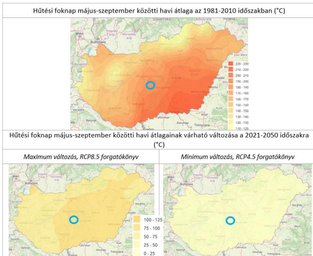
1. ábra: Hűtési célú energiaigényt befolyásoló hűtési foknap május-szeptember közötti megfigyelt és várható alakulása
