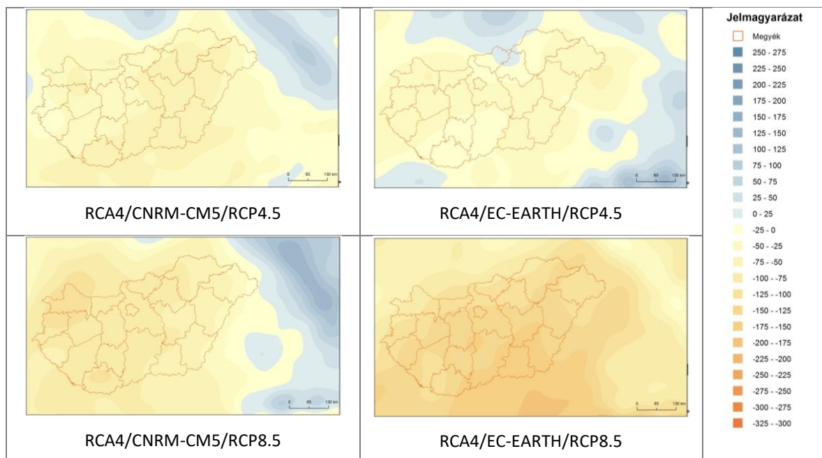
41. ábra: A klimatikus vízmérleg várható változása a Duna vízgyűjtő területén a 2071–2100 időszakra különböző klímamodell-szimulációk alapján közepesen optimista (RCP4.5) és pesszimista (RCP8.5) forgatókönyvek alapján
