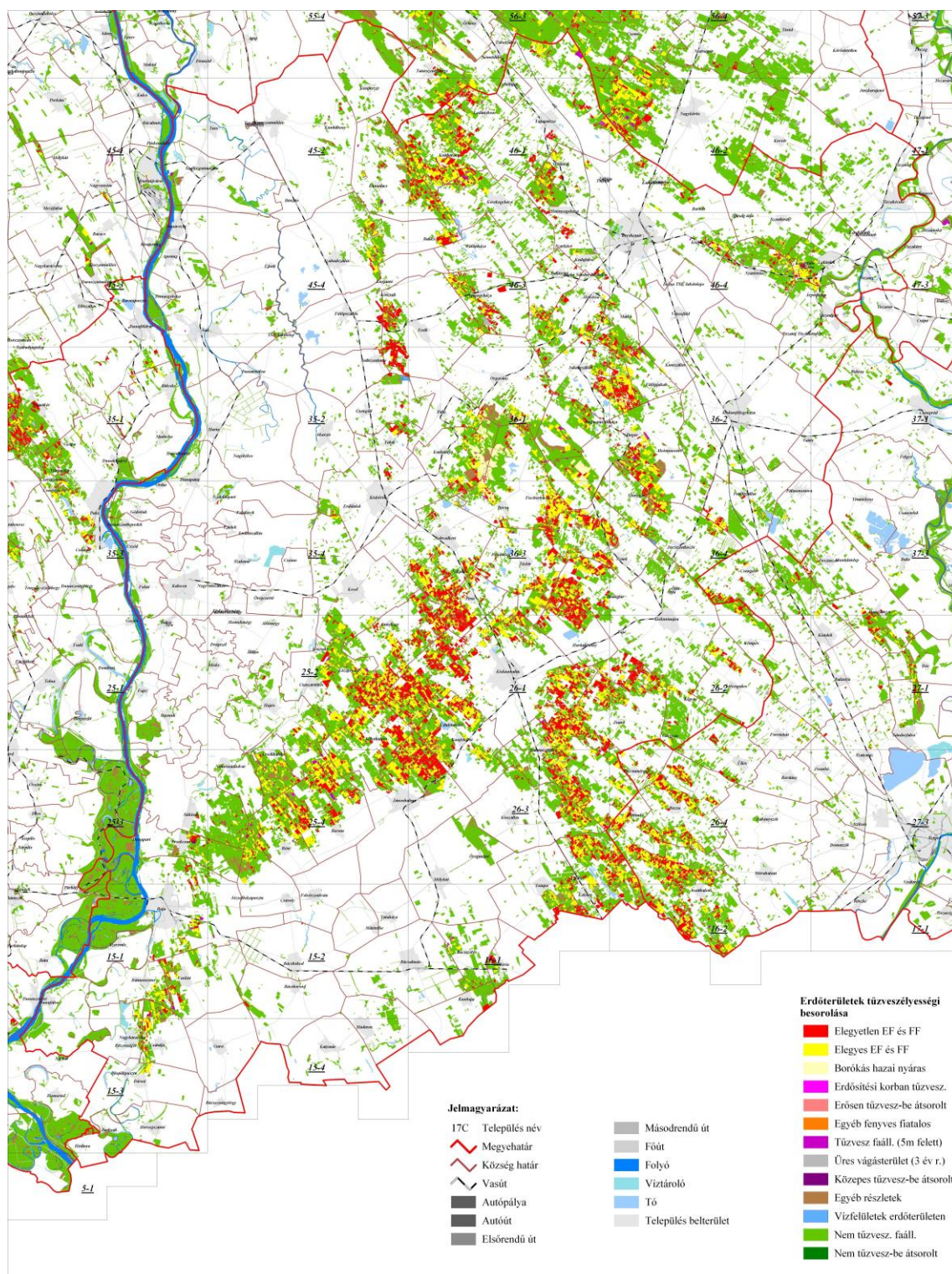
46. ábra: Bács-Kiskun vármegye Erdőtűzvédelmi terve
