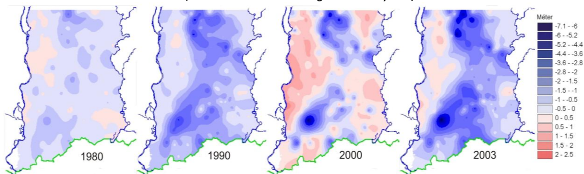
40. ábra: A talajvízszint-változás mértéke 1980, 1990, 2000 és 2003 márciusában a Duna–Tisza közén (az 1971-1975. évi átlaghoz viszonyítva)
