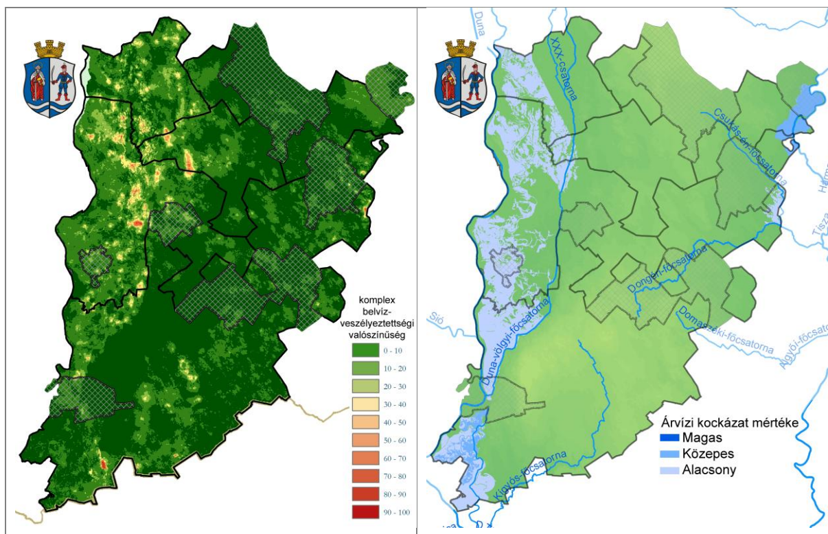
43. ábra: A Komplex Belvíz-veszélyeztetettség Valószínűség (KBV, %) területi eloszlása (bal) és az árvíz-veszélyeztetettség (jobb) Bács-Kiskun vármegyében
