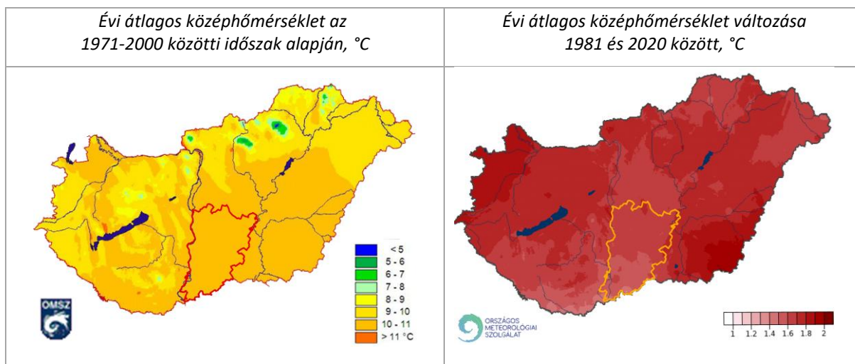
29. ábra: Évi középhőmérséklet és annak változása az elmúlt 50 évben
