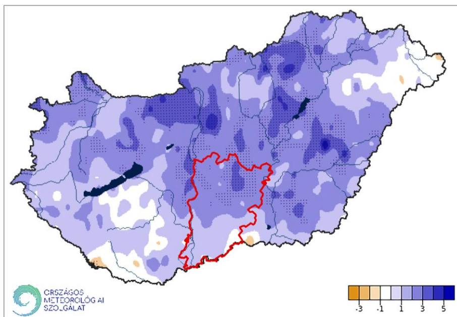
34. ábra: A nyári átlagos napi csapadékinintenzitás (átlagos csapadékoság) változása az 1981–2020 időszakban (mm/nap)
